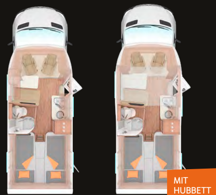
640 MEG (MB) 2-3 Personen Grundriss 640 MEG Suite (MB) 4 Personen Grundriss MIT HUBBETT
